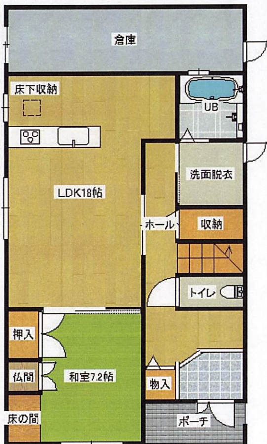
1階
